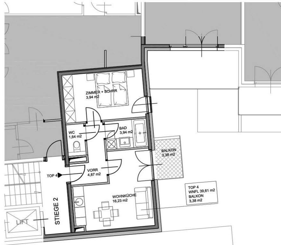
1 OBERGESCHOSS
